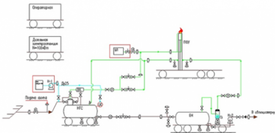
Рис. 1. Пример - принципиальная технологическая схема мобильной установки по подготовке и отгрузке нефти.
